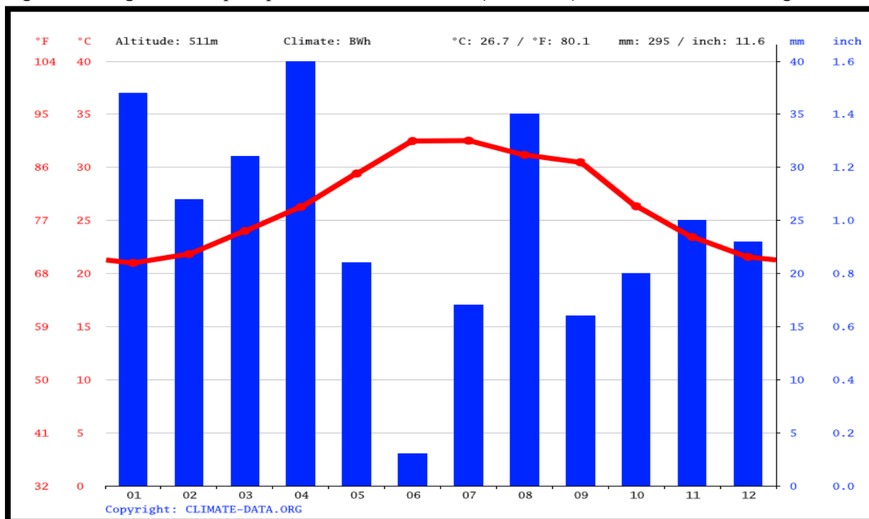
Figure 3 : Diagramme de précipitations Ali-sabieh-ville (Ali-sabieh), source : climat-data.org
