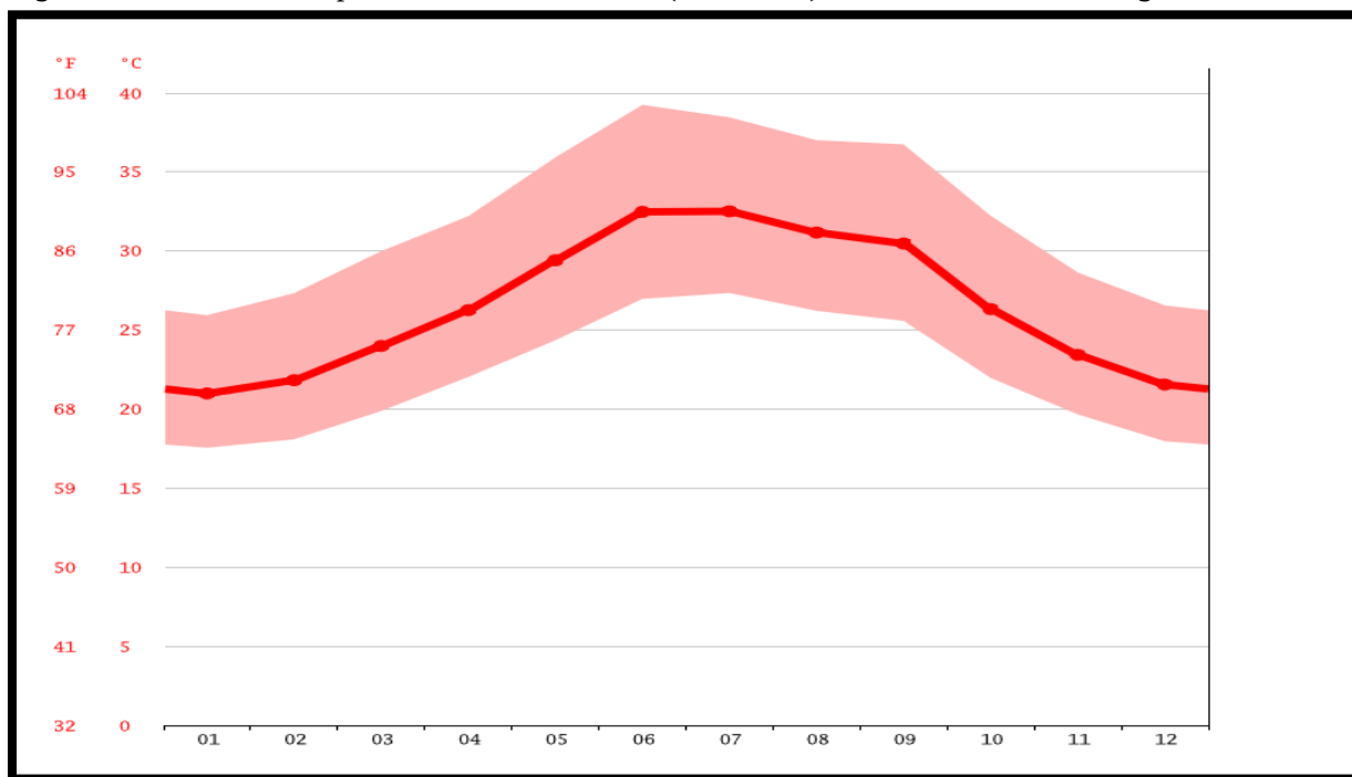
Figure 2 : Courbe de température Ali-sabieh-ville (Ali-sabieh), source : climat-data.org
