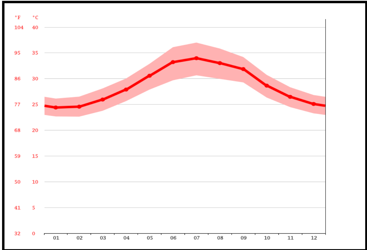
Figure 2 : Courbe de température Assassan (Obock), source : climat-data.org
