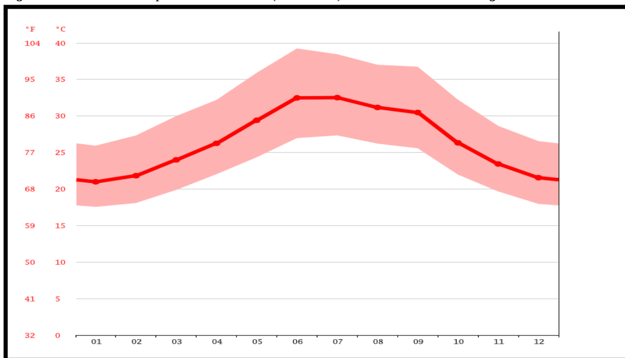
Figure 2 : Courbe de température Guelilleh (Ali-sabieh), source : climat-data.org
