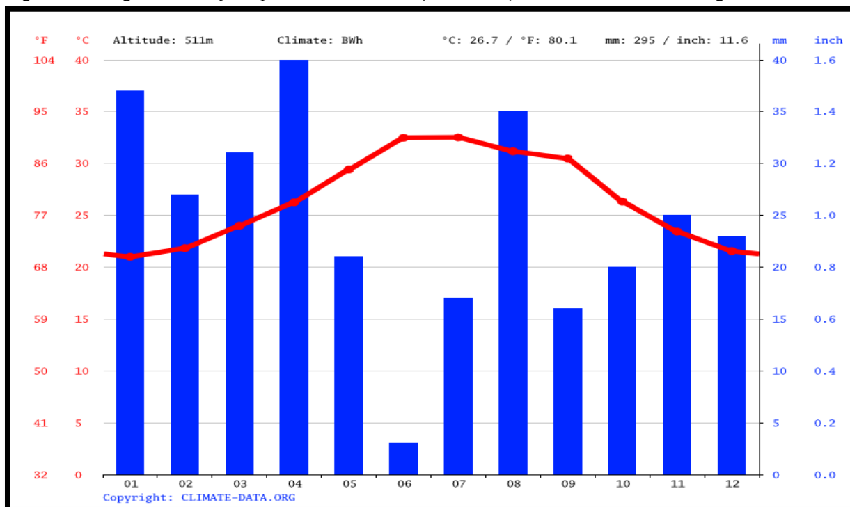
Figure 3 : Diagramme de précipitations Guelilleh (Ali-sabieh), source : climat-data.org
