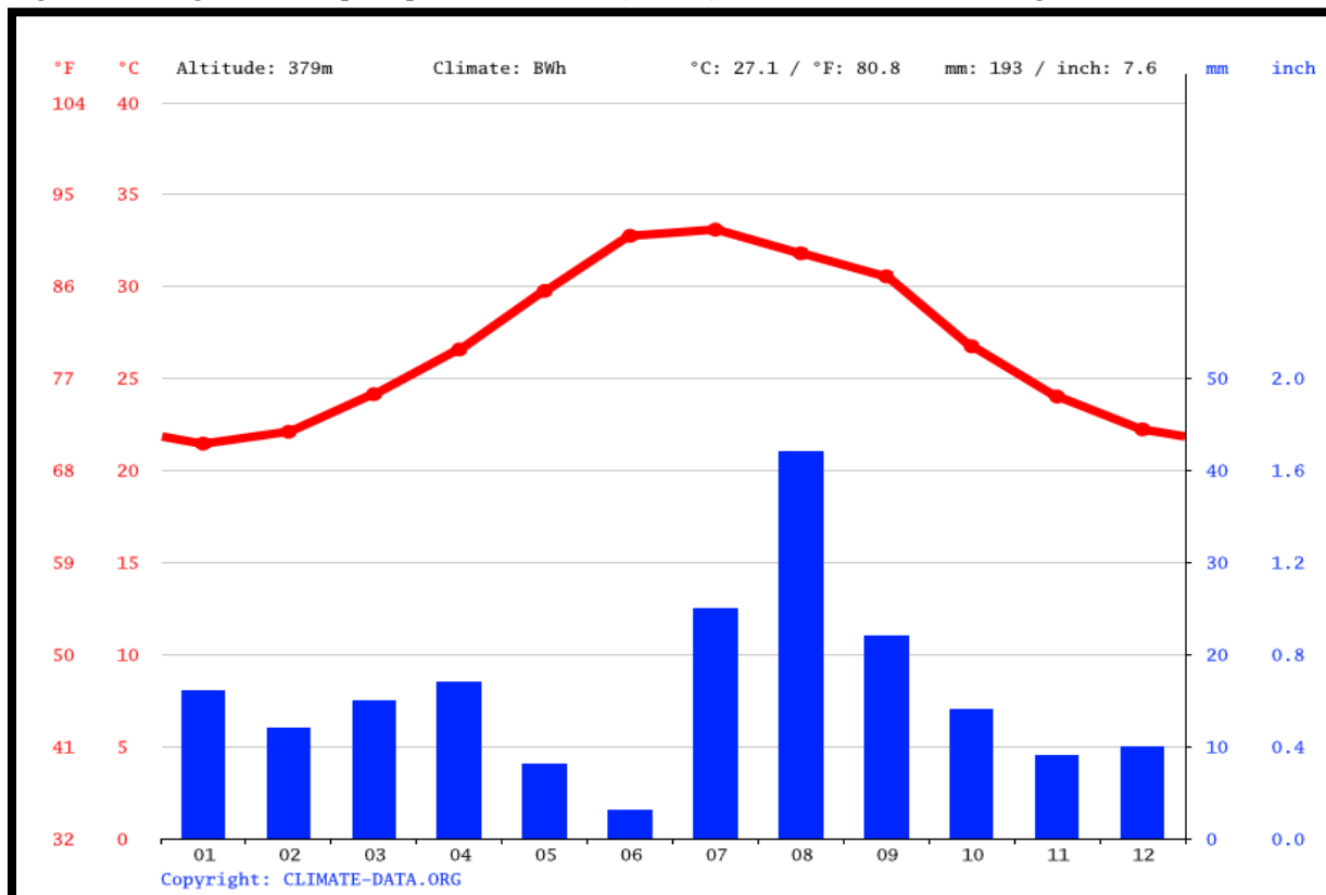
Figure 3 : Diagramme de précipitations Waddi (Obock), source : climat-data.org
