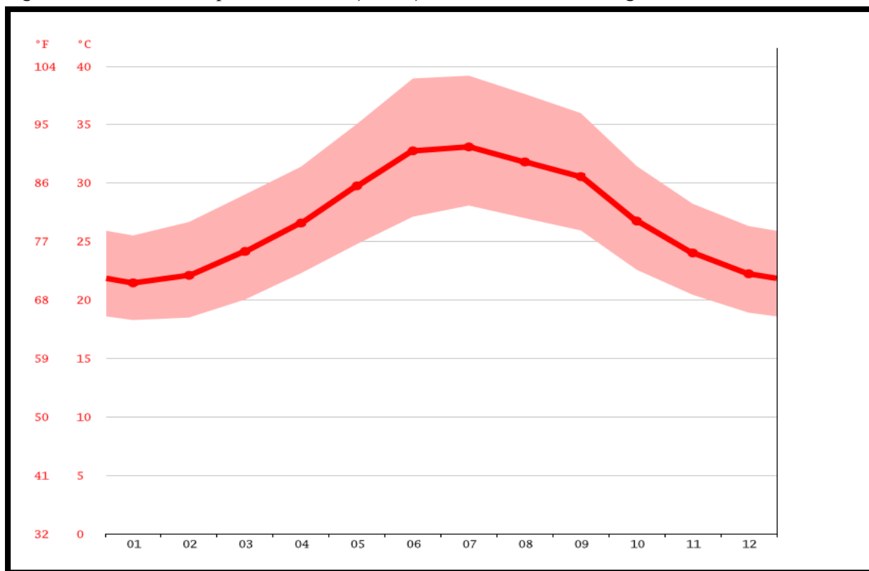
Figure 2 : Courbe de température Waddi (Obock), source : climat-data.org
